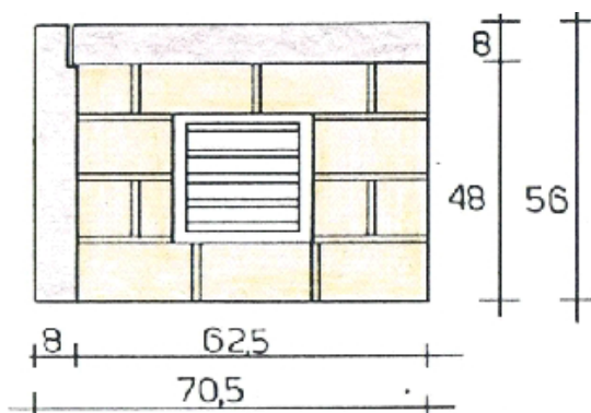
PIANTA
