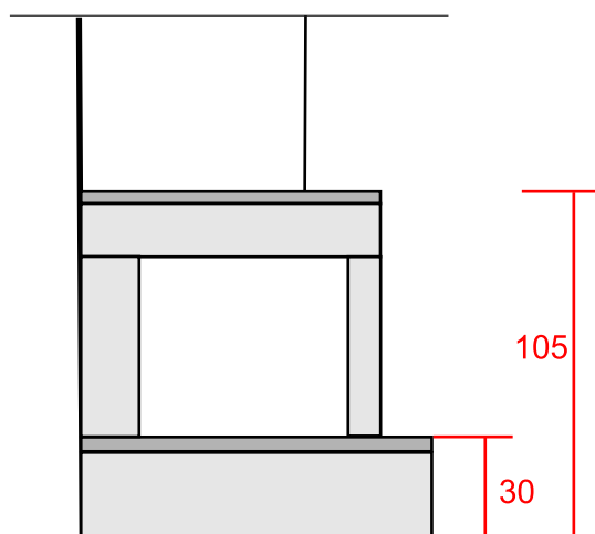
PROSPETTO
