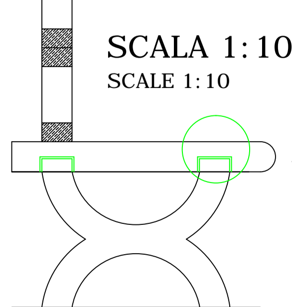
PARTICOLARE COSTRUTTIVO SCHIENALE/PIEDE CONSTRUCTION DETAIL BACK / SUPPORT
