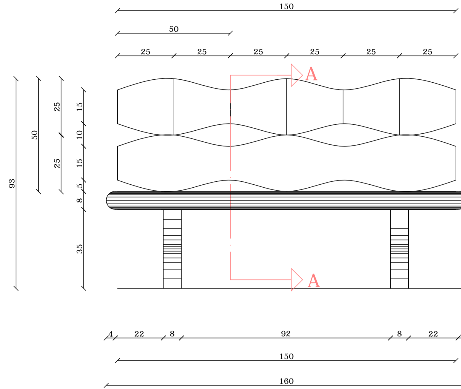
PROSPETTO FRONTALE SCALA 1:10 ELEVATION FRONT SCALE 1:10
