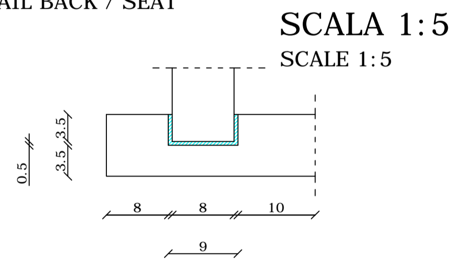
PARTICOLARE COSTRUTTIVO SCHIENALE/SEDUTA CONSTRUCTION DETAIL BACK / SEAT
