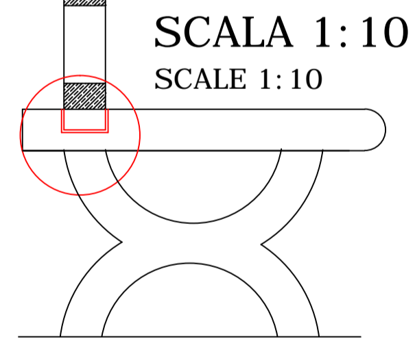
PARTICOLARE COSTRUTTIVO SCHIENALE/SEDUTA CONSTRUCTION DETAIL BACK / SEAT
